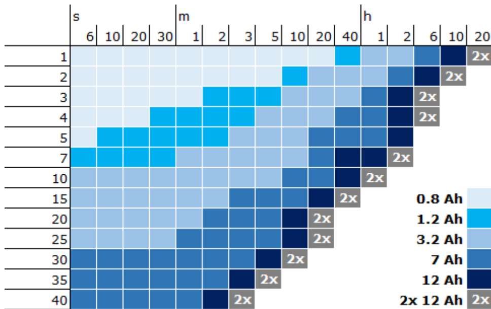
Abbildung 10: Pufferzeit in Abhängigkeit des Laststroms
