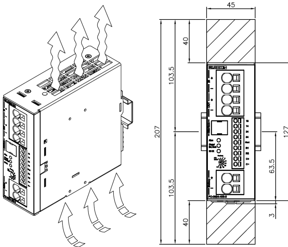
Abbildung 5: Konvektionskühlung
