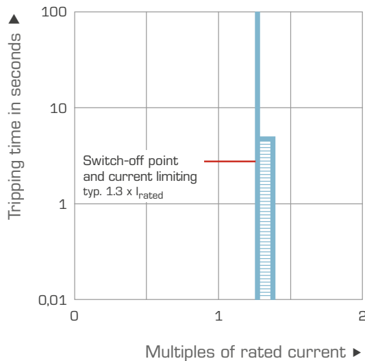
Auslösekennlinie PM-2824-xxx-x
