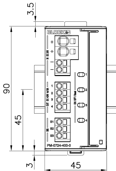
Abmessungen 4/2-Kanal-Module
