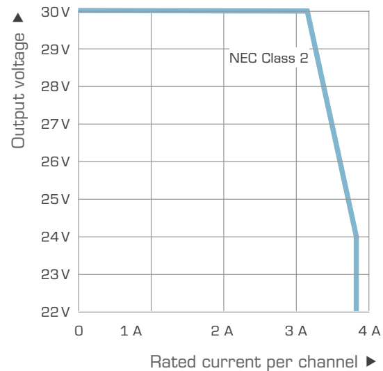
Auslösekennlinie PM-9824-xxx-x
